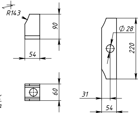
Поз.4 (Ушко)
