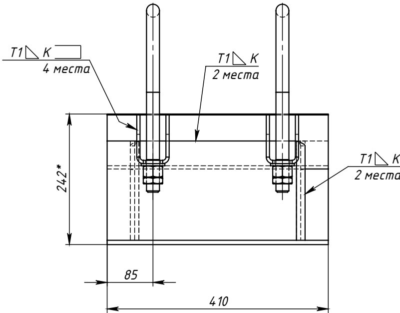
Поз.1 (Ложемент)
