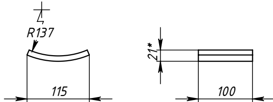
Поз.6 (Упор)
