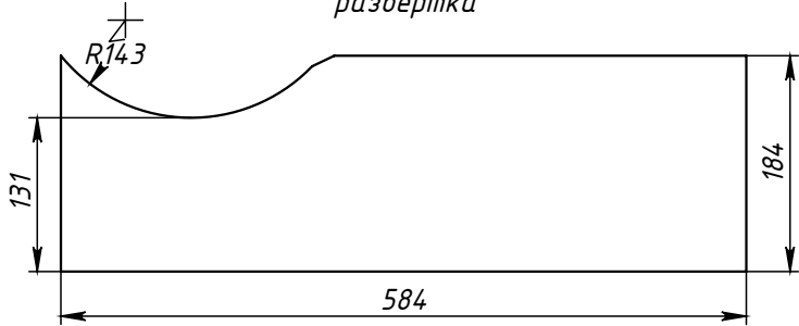
Поз.3 (Угольник) развертка
